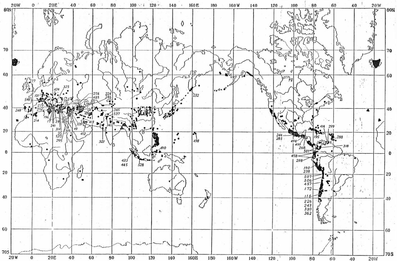
地第 29 図 世界大地震分布図 (太古から 1899 年まで)
